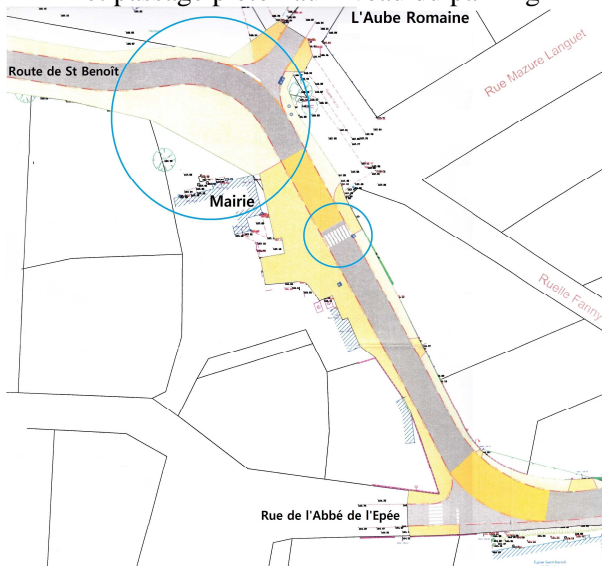
Réaménagement du virage de la mairie et passage piéton au niveau du parking
