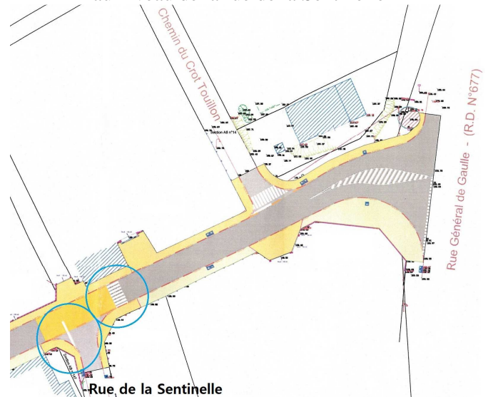
Passage piéton et cédez le passage au niveau de la rue de la Sentinelle
